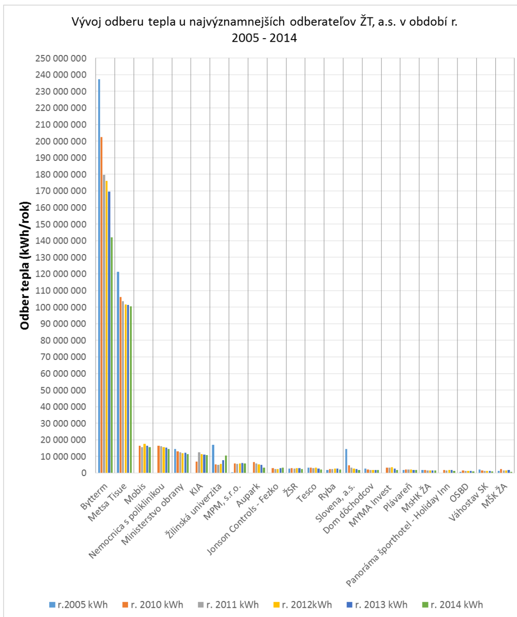
Obr. 63 Vývoj odberu tepla najvýznamnejších odberateľov Žilinskej teplárenskej v rokoch 2005, 2010 - 2014
